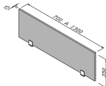
Painel Divisor Suspenso MDP 15mm Cód: PNDV120/ PNDV140/ PNDV160 Medidas: L 700 a 1300 x P 15 x A 350mm.
