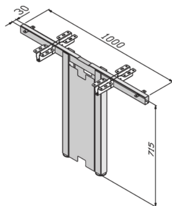
Estrutura Central Shaft - Frente e Verso Tubo 50x50 Cód: ESTC1400CS Medidas: L 30 x P 1000 x A 715mm.
