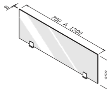
Painel Divisor Suspenso em Vidro Transparente/ Colorido/ Jateado Cód: PNV120T/ PNV140T/ PNV160T - Transparentes PNV120C/ PNV140C/ PNV160C - Coloridos PNV120J/ PNV140J/ PNV160J - Jateados Medidas: L 700 a 1300 x P 8 x A 350mm.
