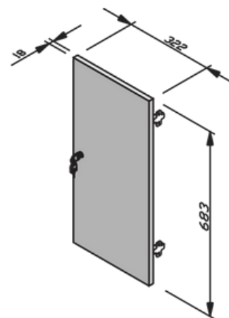
Porta Alta Para Armário Complemento Cód: ? Medidas: L 322 x P 18 x A 683mm.
