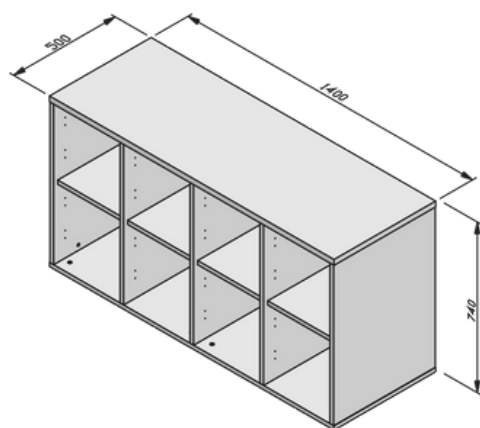
Armário Complemento Plataforma Easy com Portas Modulares Cód: FT077N Medidas: L 1400 x P 500 x A 740mm.
