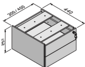
Gaveteiro Fixo 2 Gavetas Gaveta em Aço Cód: GVPL010 Medidas: L 300 e 400 x P 440x A 257mm.
