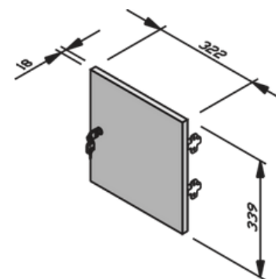
Porta Baixa Para Armário Complemento Cód: ? Medidas: L 322 x P 18 x A 339mm.
