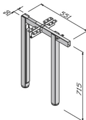
Estrutura Central Lado a Lado Tubo 50 x 50mm - Sem Shaft Cód: ESTC700C Medidas: L 50 x P 551 x A 715mm.
