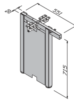
Estrutura Central Shaft - Lado a Lado Tubo 50 x 50mm - Com Shaft Cod: ESTC700CS Medidas: L 50 x P 551 x A 715mm.
